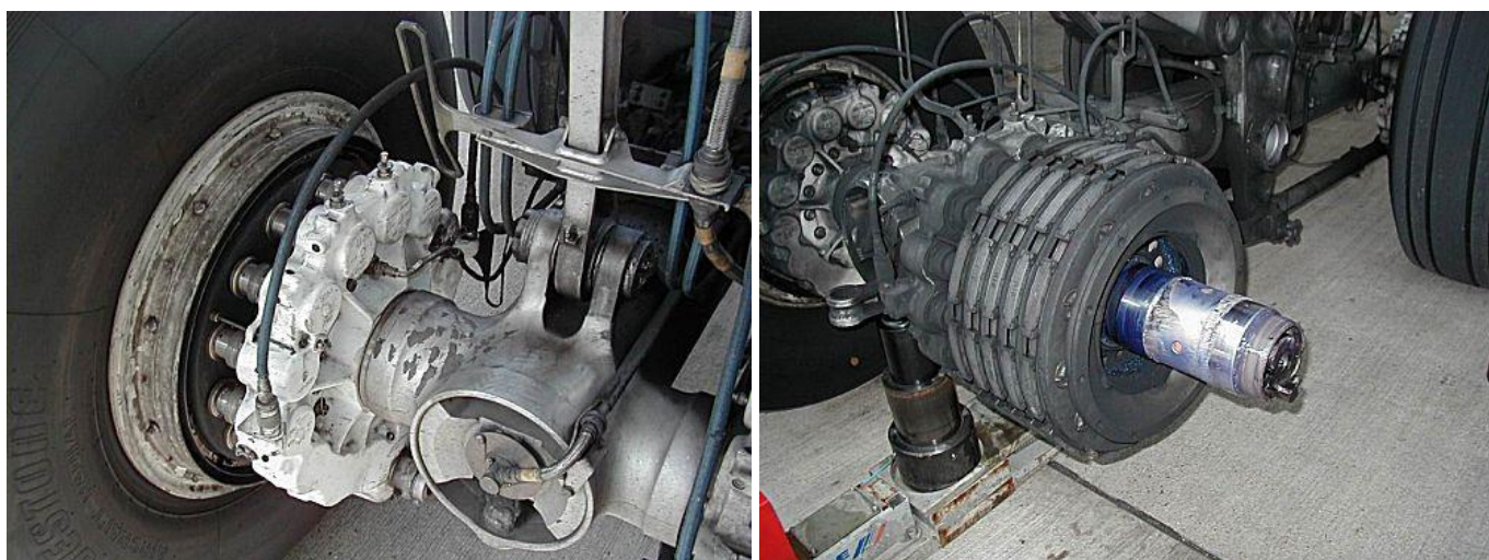
Train A340, freinage hydraulique conventionnel
