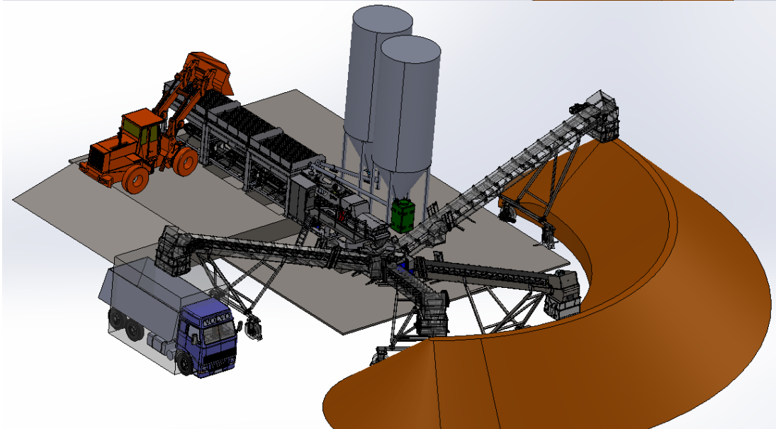
Plan projet 3D sous SOLIDWORKS
