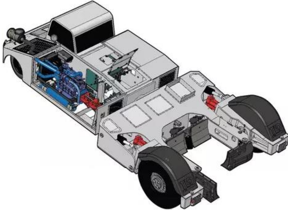
Tracteur towbarless TPX500S
